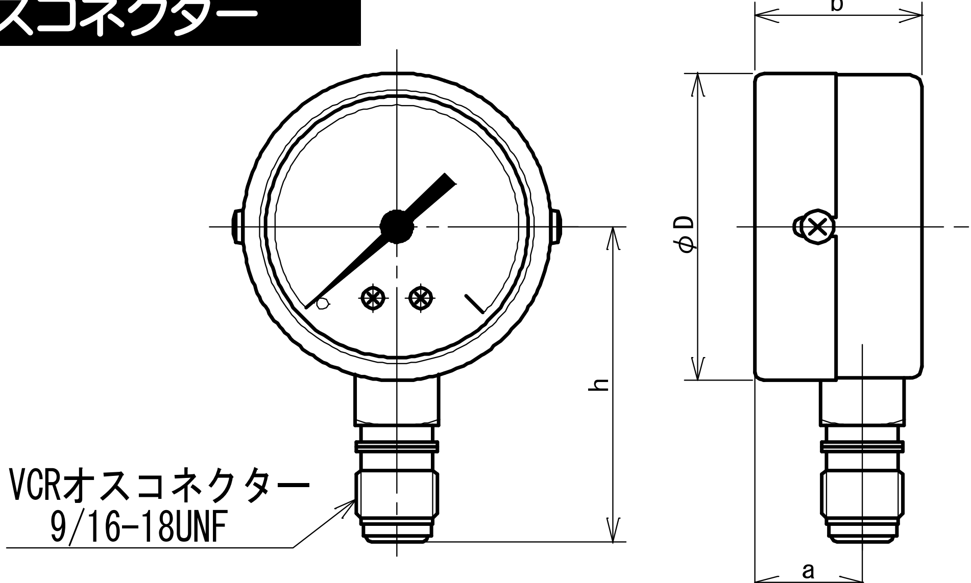
A形VCRオスコネクター
