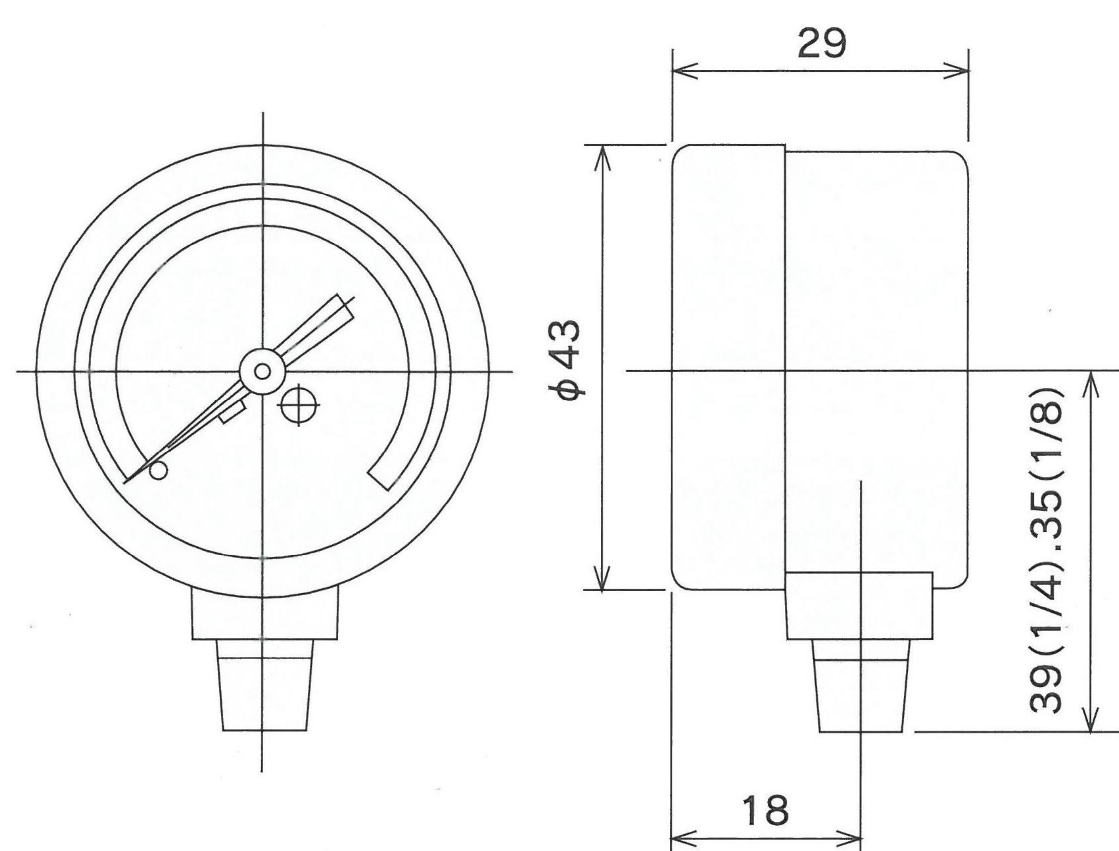
A40形
